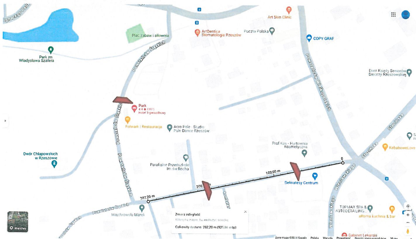
Rysunek 1. Odcinek 300m do wykonania całościowej nakładki asfaltowej oraz propozycja progów spowalniających po wykonaniu całościowej nakładki asfaltowej
